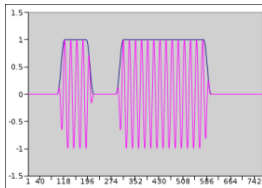
Figure 2.115 Dash/Dot = 3.0, Edge = 3 msec
