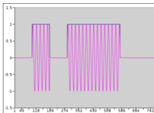
Figure 2.113 Dash/Dot = 3.0, Edge = 0.0
